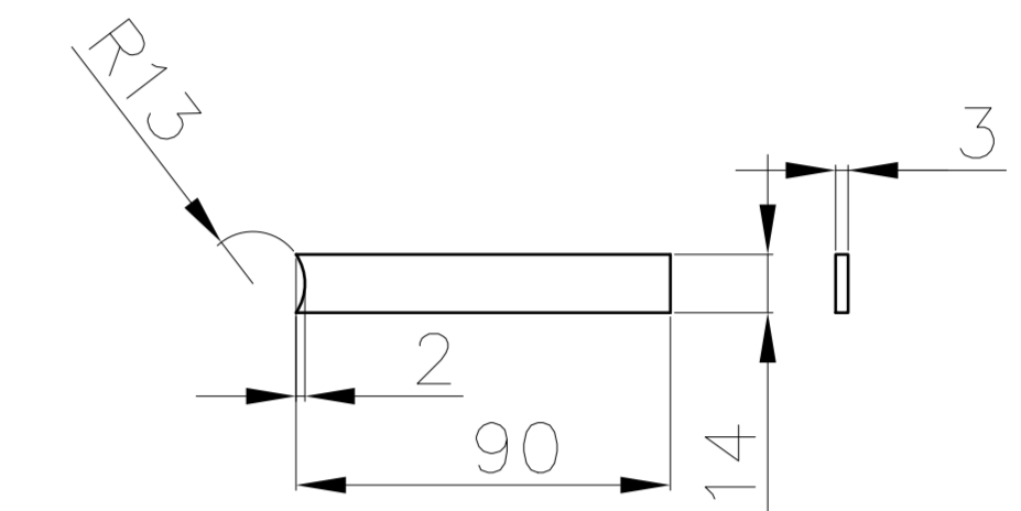
Rys.671/5
