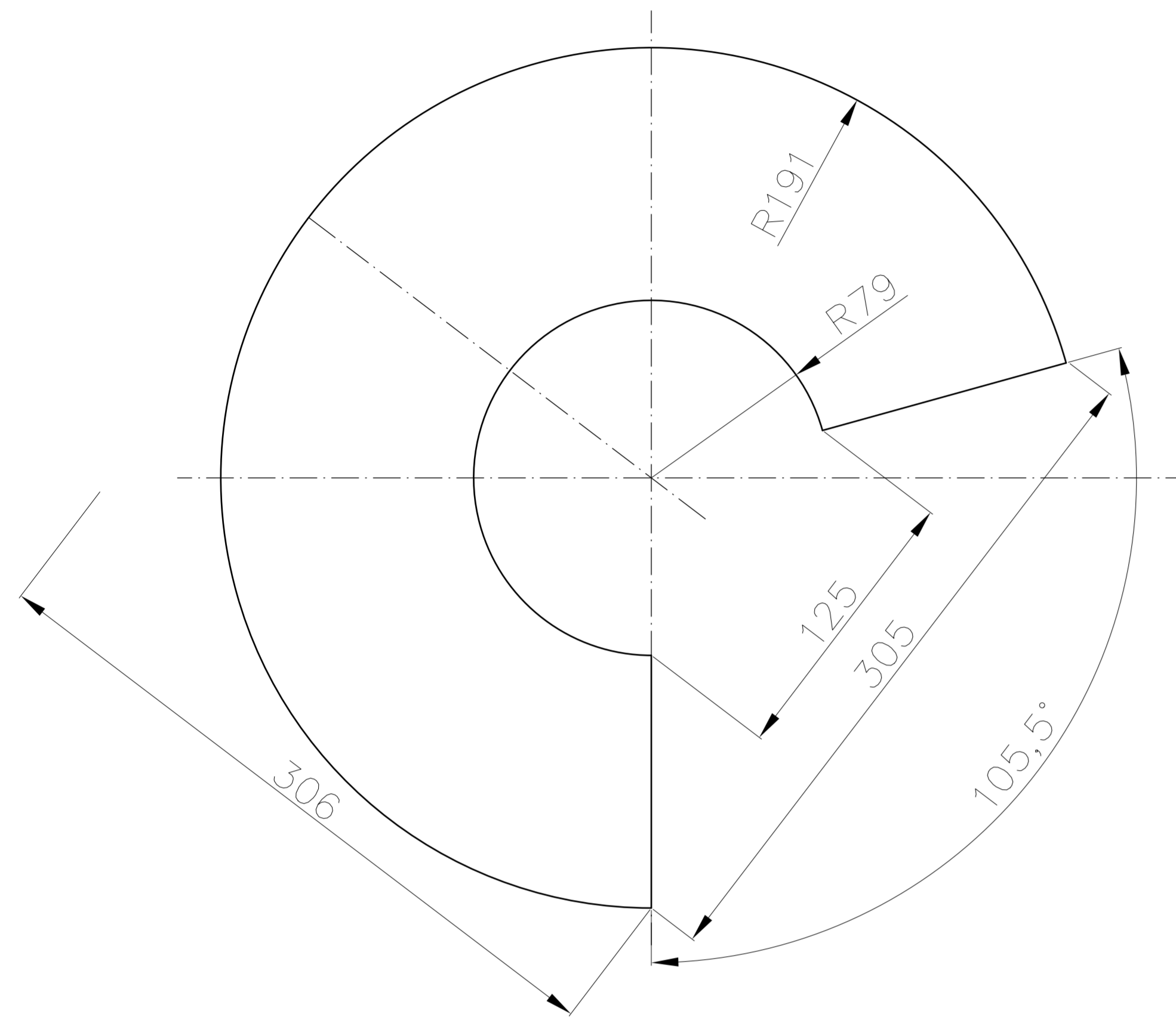
Rys.671/1
