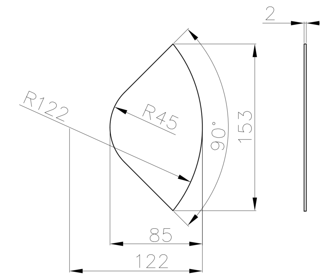
Rys.671/4
