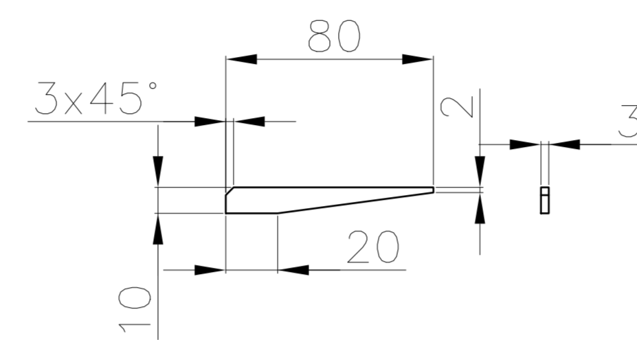
Rys.671/3
