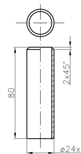
Rys.673/77
