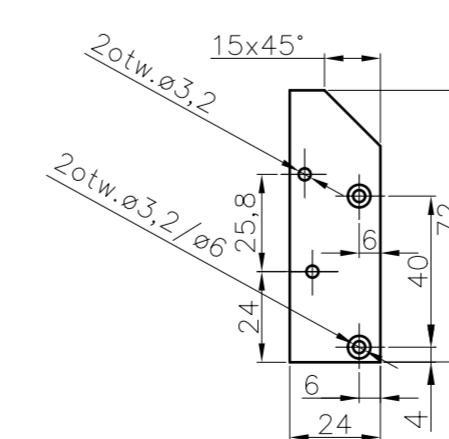
Rys.673/78
