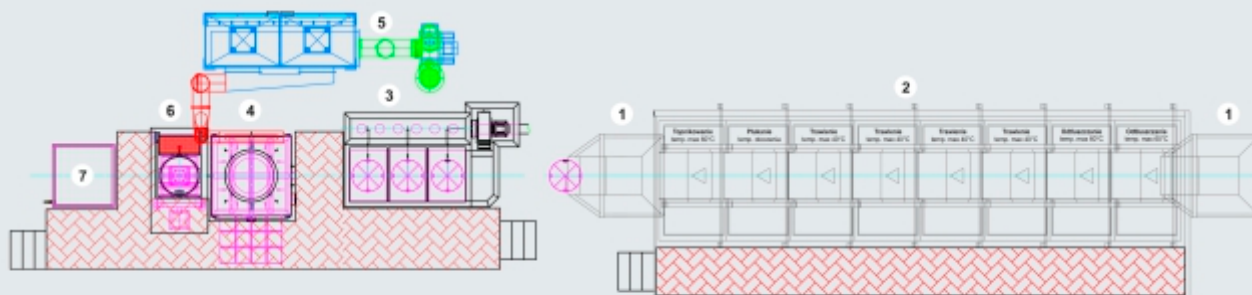
OPIS: 1. Wibracyjny zbiorniki dozujący; 2. Linia przygotowania powierzchni; 3. Suszarka; 4. Piec; 5. Filtr; 6. Wirówka; 7. Wanna wodna
